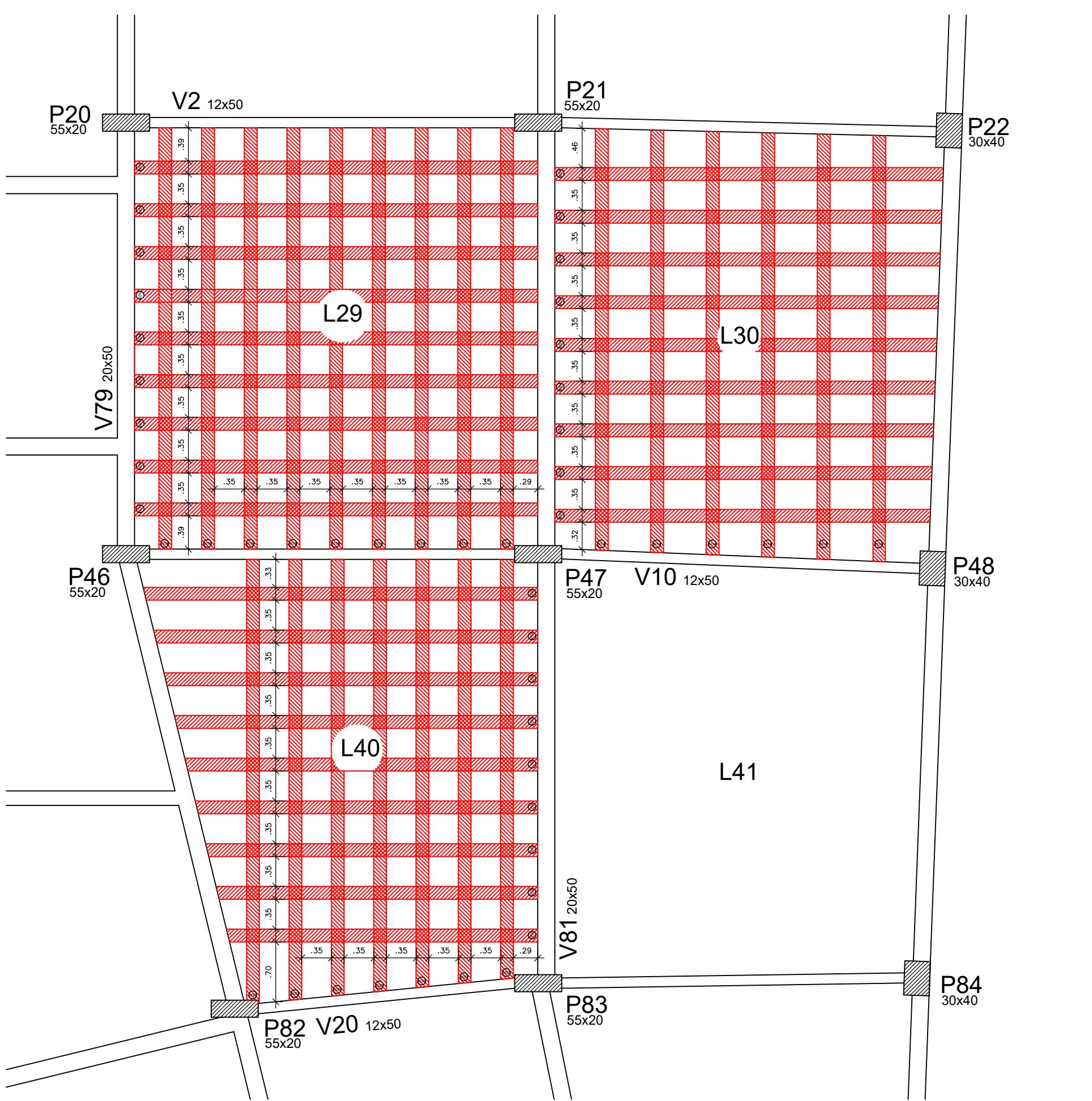
PLANO DE CORTE DAS MANTAS DE FIBRA DE CARBONO
