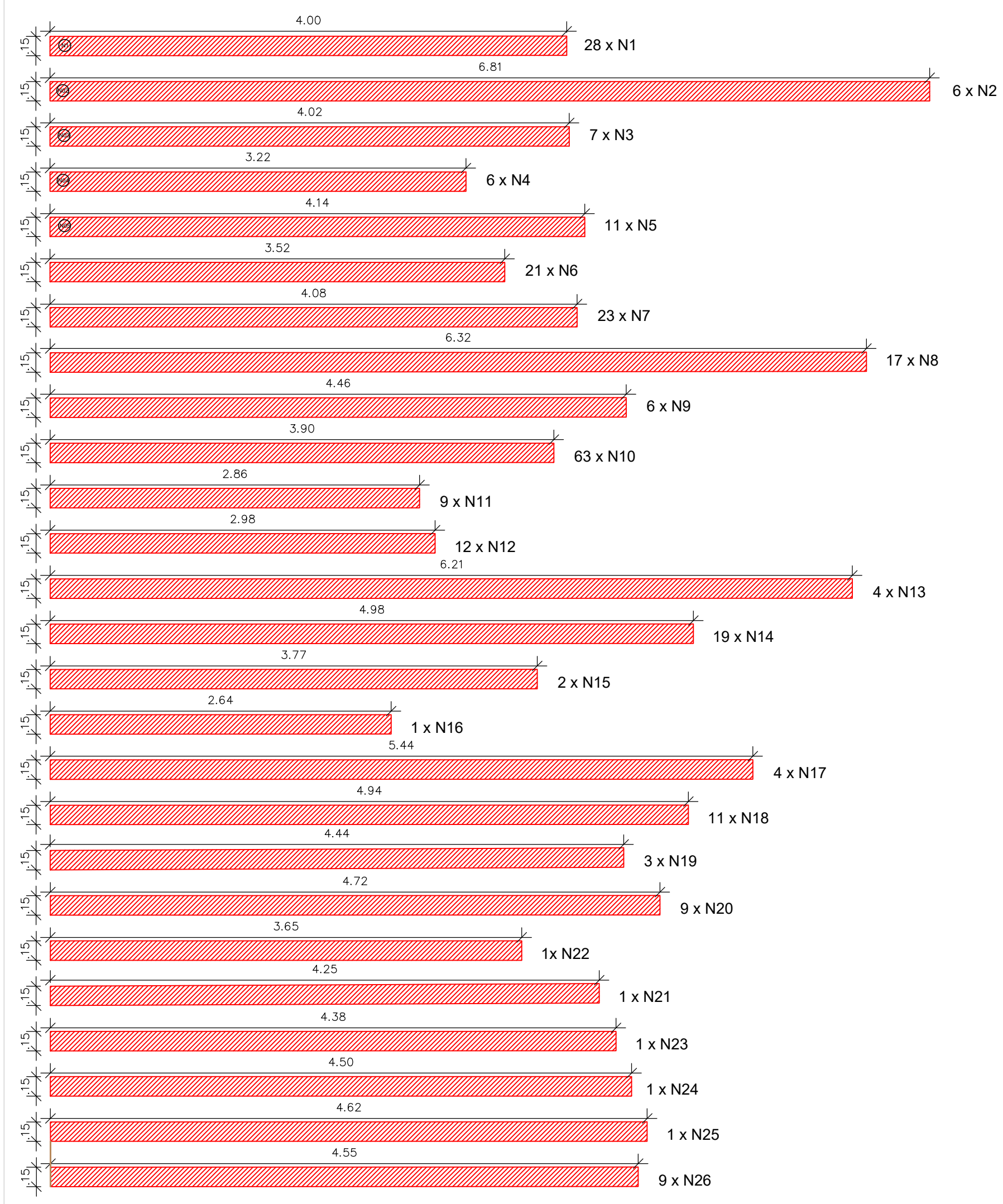
PLANO DE CORTE DAS MANTAS DE FIBRA DE CARBONO
